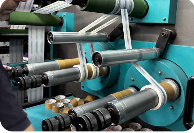
Üst Baskı Makinesi
